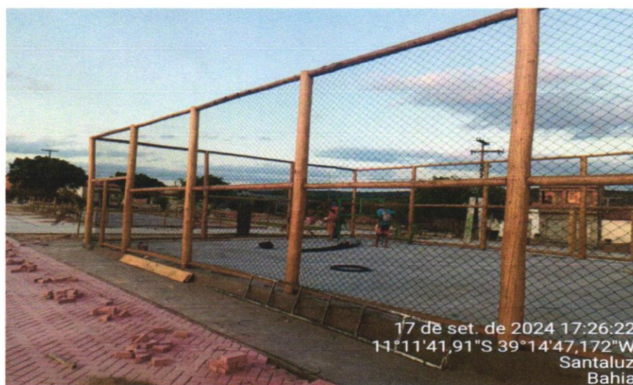
FOTO 2: ALAMBRADO PARA QUADRA POLIESPORTIVA, ESTRUTURADO POR TUBOS DE AÇO GALVANIZADO, (MONTANTES COM DIAMETRO 2", TRAVESSAS E ESCORAS COM DIÂMETRO 1 ¼), COM TELA DE ARAME GALVANIZADO, FIO 10 BWG E MALHA QUADRADA 5X5CM (EXCETO MURETA). AF_03/202
